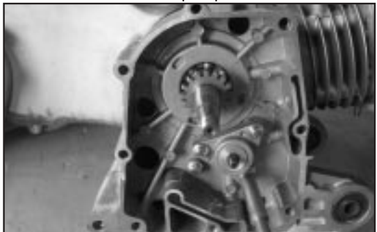
Zahnrad des Ölpumpenantriebs Befestigungs- Ölpumpe klemmen
